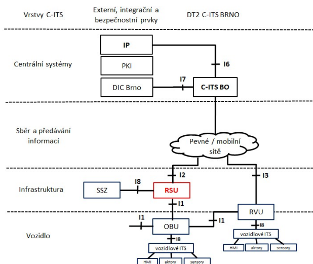
Obrázek 39 Architektura umístění a napojení RSU jednotek
