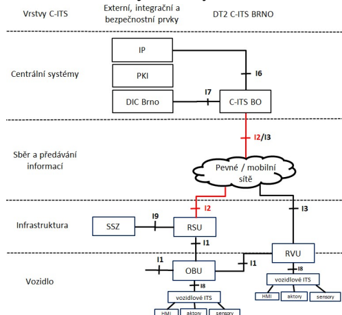
Obrázek 32 Architektura systému vč. rozhraní I2
