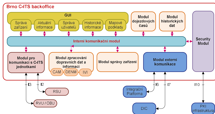
Obrázek 27 Funkční architektura C-ITS back office
