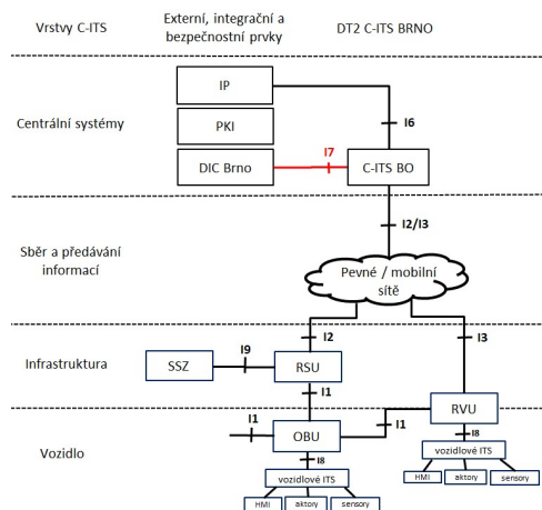
Obrázek 35 Architektura systému vč. rozhraní I7
