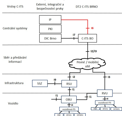
Obrázek 34 Architektura systému vč. rozhraní I6
