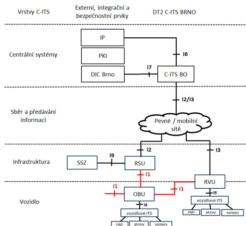
Obrázek 28 Architektura umístění a napojení rozhraní I1
