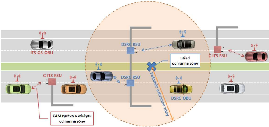
Obrázek 26 Příklad koexistence mezi ITS-G5 a CEN-DSRC
