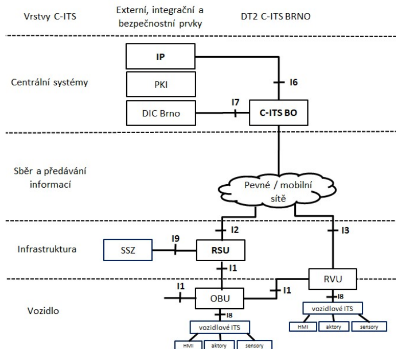
Obrázek 1 Architektura C-ITS systému ve městě Brně
