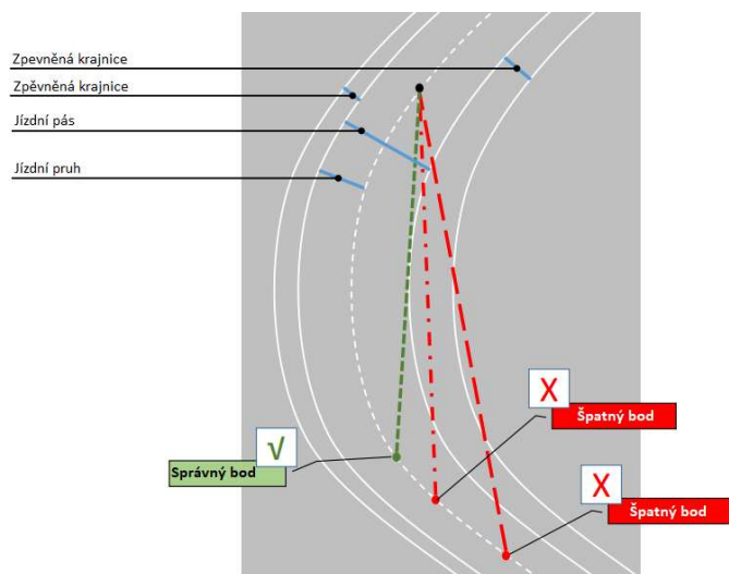
Obrázek 22 Umístění bodů Traces ve směrovém oblouku
