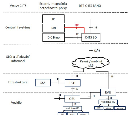
Obrázek 38 Architektura systému vč. rozhraní I10
