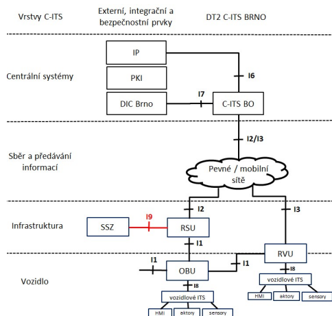
Obrázek 37 Architektura systému vč. rozhraní I9
