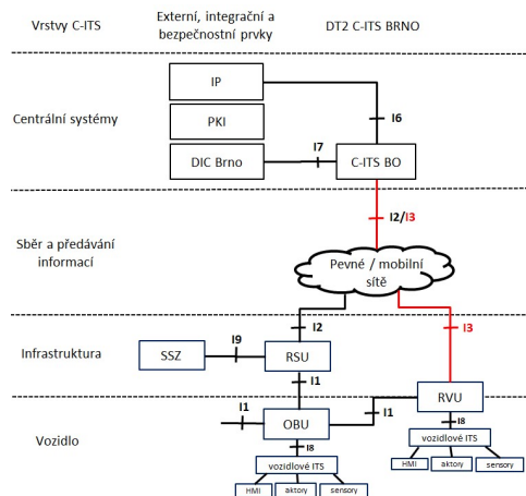
Obrázek 33 Architektura systému vč. rozhraní I3
