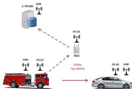
Obrázek 3 Schéma fungování služby EVA – mobilní režim
