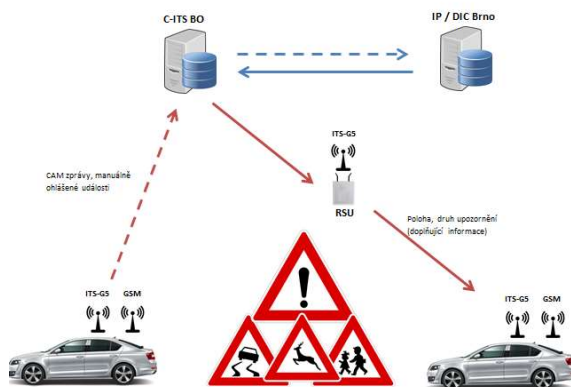
Obrázek 14 Schéma fungování služby HLN
