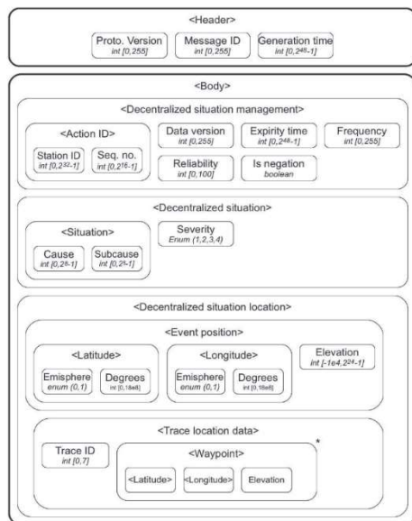
Obrázek 30 Struktura zprávy DENM
