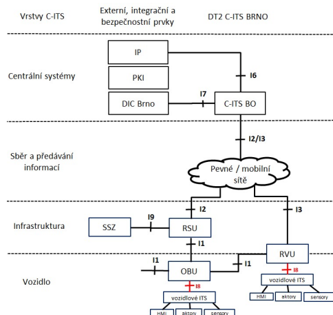
Obrázek 36 Architektura systému vč. rozhraní I8
