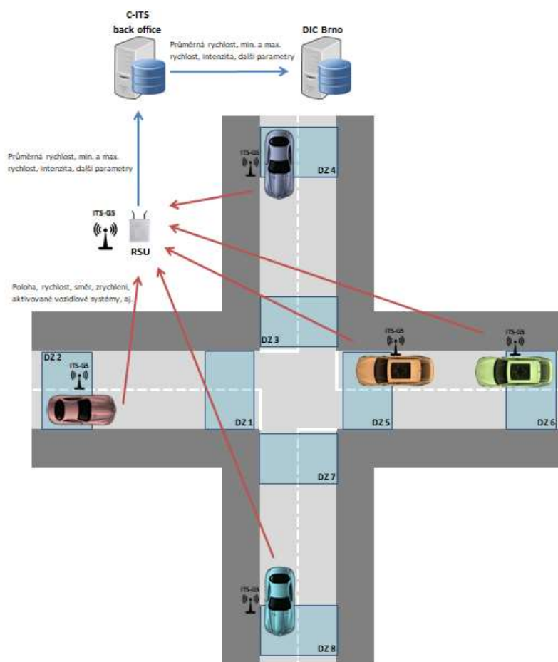
Obrázek 2 Schéma fungování služby PVD
