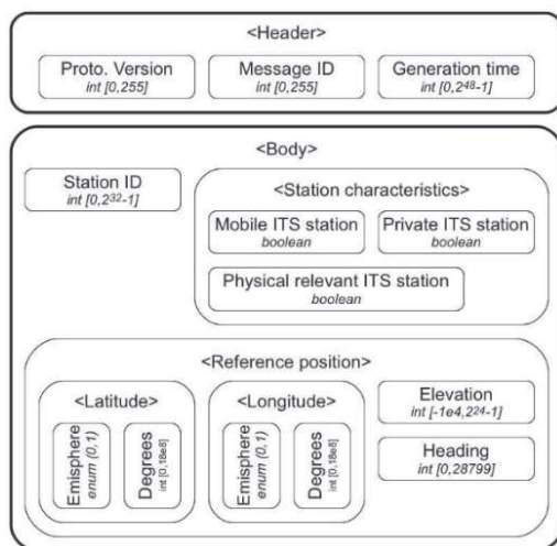
Obrázek 29 Struktura zprávy CAM
