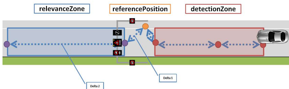
Obrázek 24 Princip vytváření bodů atributu Zones
