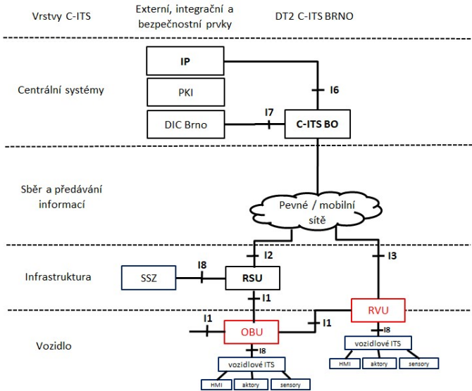
Obrázek 41 Architektura umístění a napojení vozidlových jednotek (OBU/RVU)
