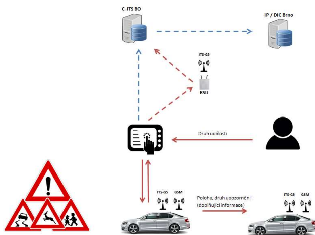
Obrázek 17 Schéma fungování služby HLN - Generování ve vozidle
