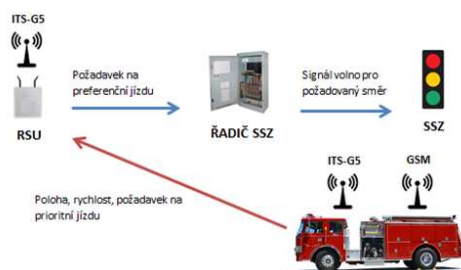
Obrázek 5 Schéma fungování služby EVA – Preference vozidel IZS
